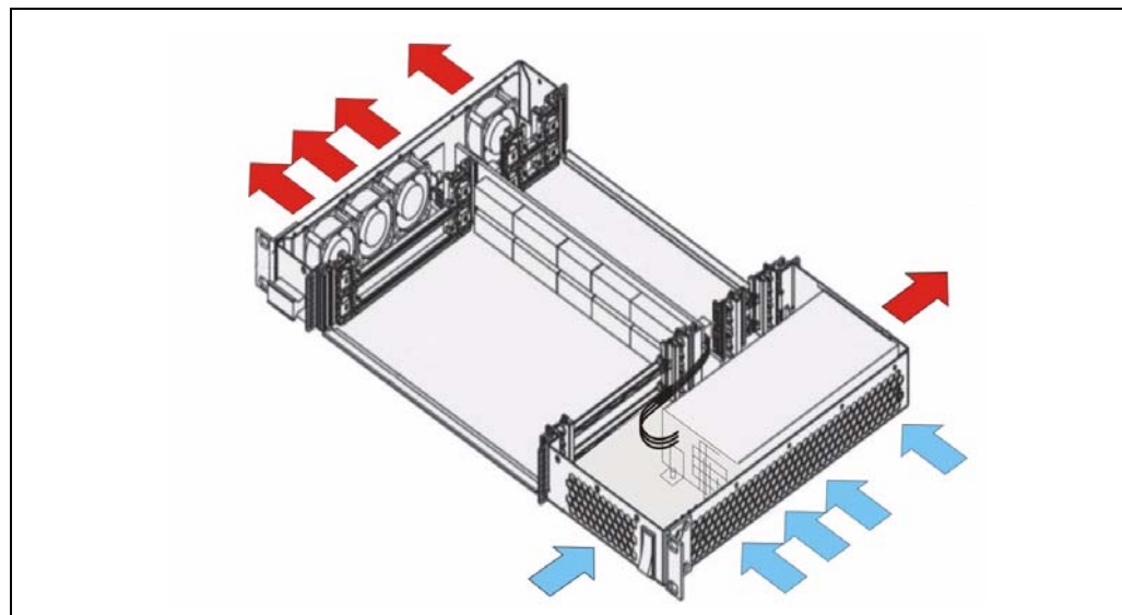
Figure 4: Entwärmung
